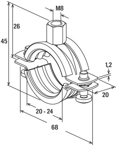
Maßzeichnung
