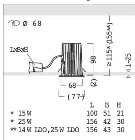
Maßzeichnung
