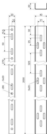
Maßzeichnung
