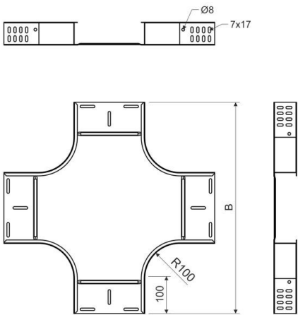
Maßzeichnung
