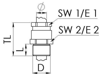
Maßzeichnung
