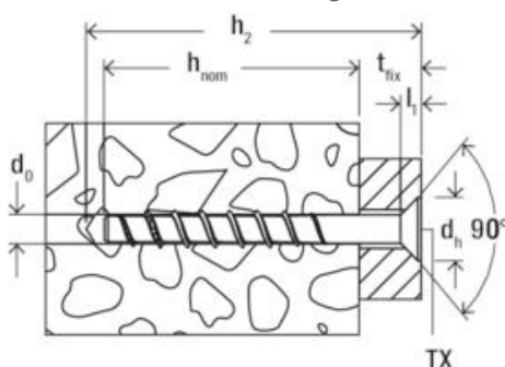
Strichzeichnung
