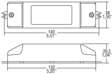
Maßzeichnung
