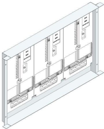
Zählerwanne mit Zählerplatte
