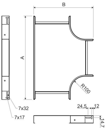
Maßzeichnung
