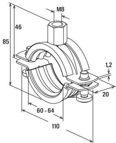
Maßzeichnung
