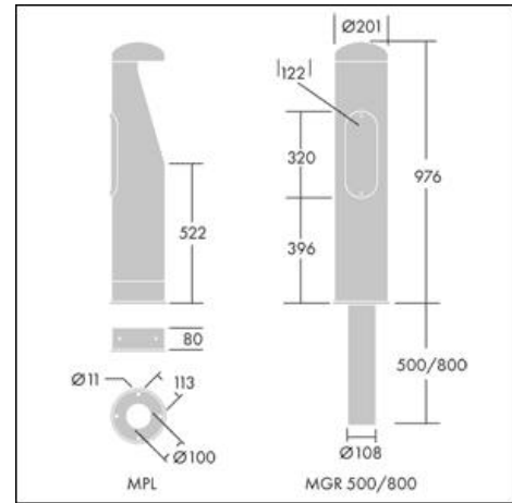
Maßzeichnung
