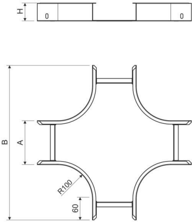
Maßzeichnung
