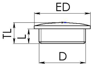
Maßzeichnung
