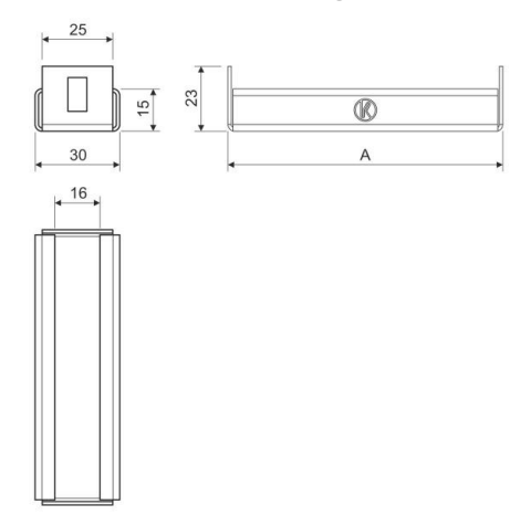
Maßzeichnung
