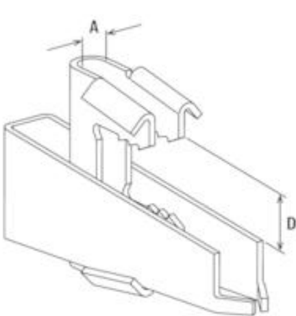
Strichzeichnung
