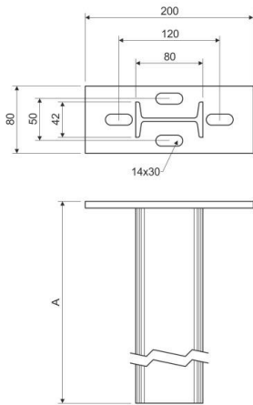
Maßzeichnung
