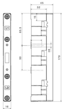
Maßzeichnung
