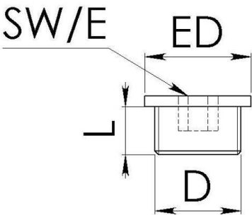
Maßzeichnung
