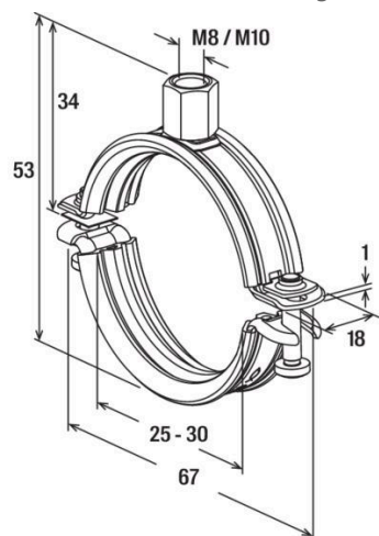
Maßzeichnung
