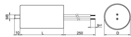
Maßzeichnung
