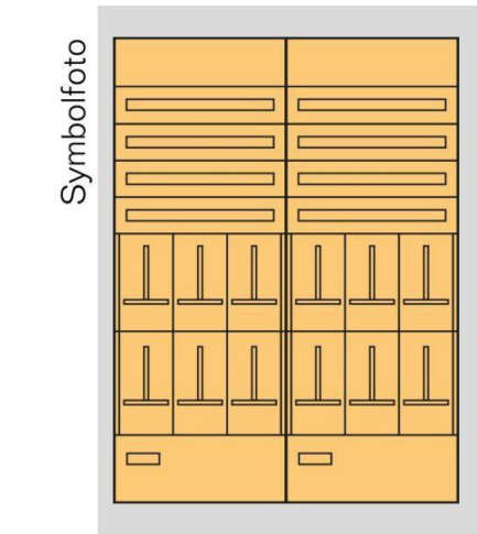
Zählerverteilereinsatz Tirol
