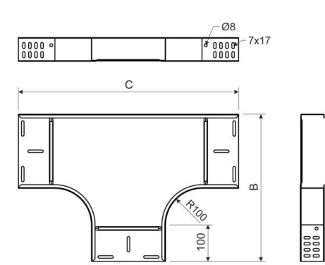
Maßzeichnung
