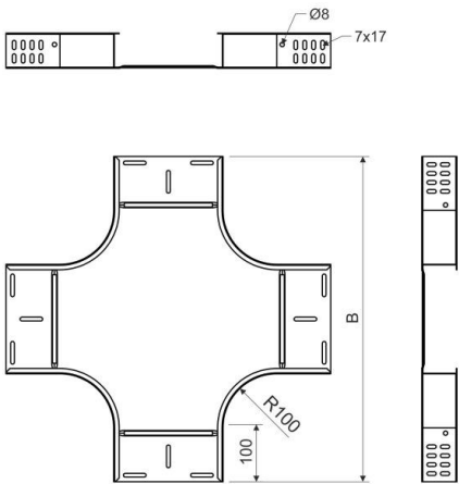
Maßzeichnung
