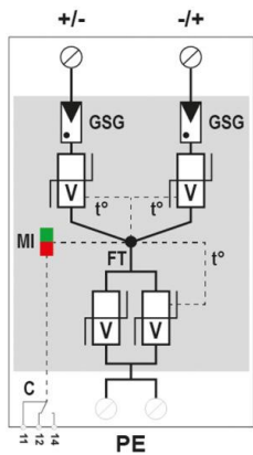
Schaltbild
