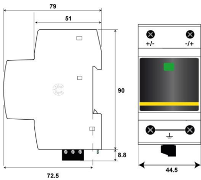
Maßzeichnung
