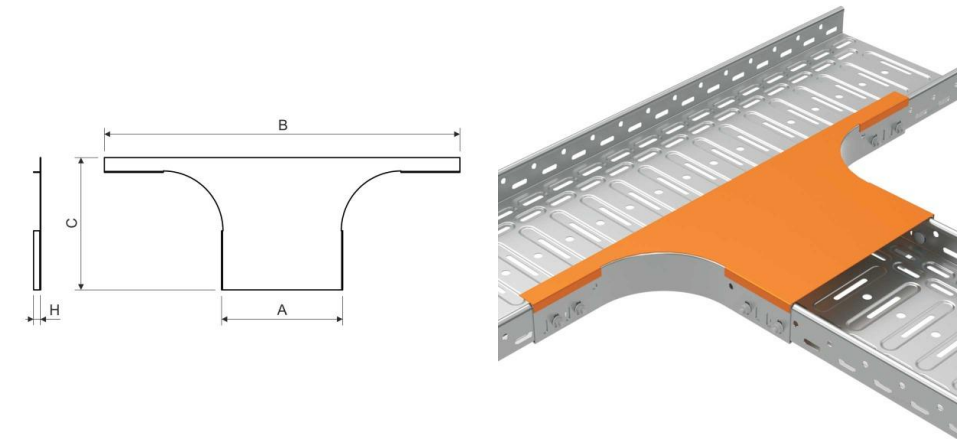
Maßzeichnung
