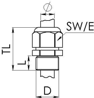
Maßzeichnung
