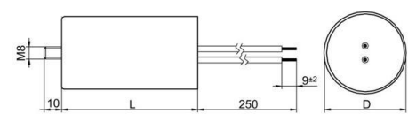
Maßzeichnung
