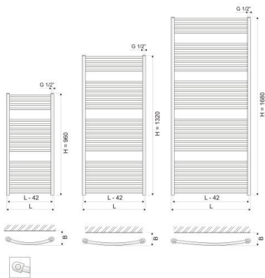
Maßzeichnung
