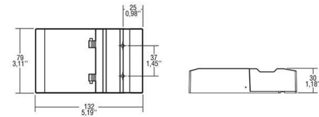
Maßzeichnung
