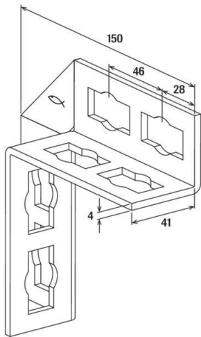
Maßzeichnung
