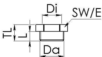
Maßzeichnung
