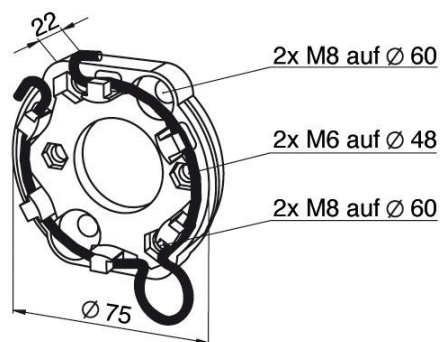
Maßzeichnung
