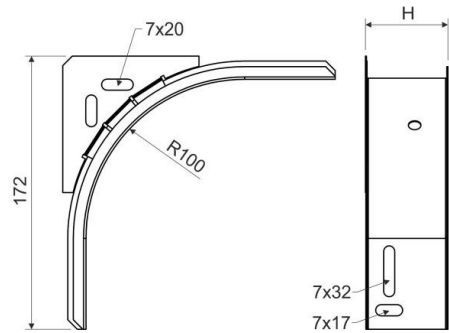
Maßzeichnung
