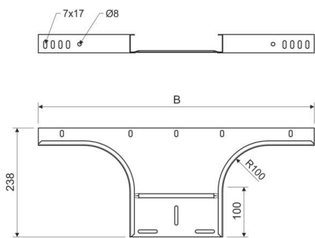
Maßzeichnung
