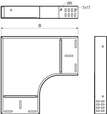
Maßzeichnung
