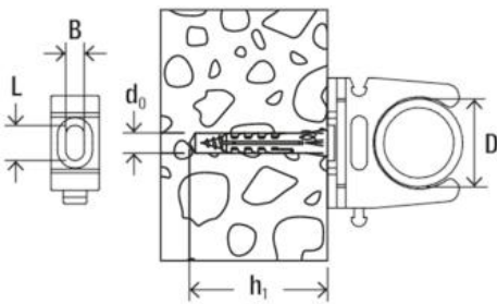
Strichzeichnung
