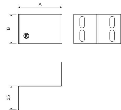
Maßzeichnung
