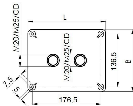
Maßzeichnung
