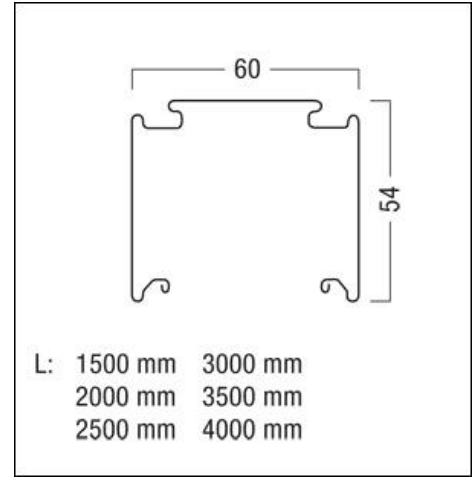
Maßzeichnung
