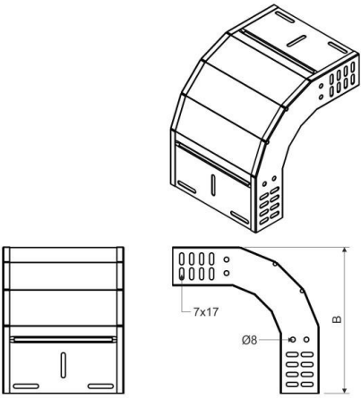
Maßzeichnung
