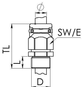
Maßzeichnung
