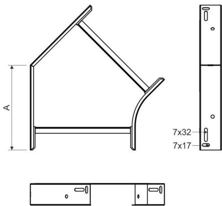
Maßzeichnung
