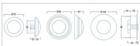
Maßzeichnung
