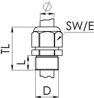
Maßzeichnung
