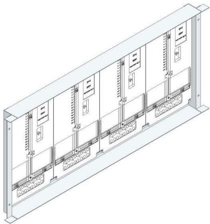
Zählerwanne mit Zählerplatte
