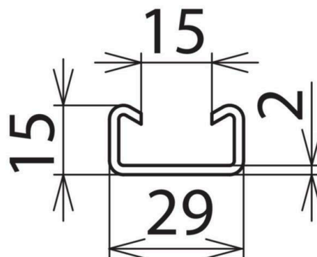
Maßzeichnung
