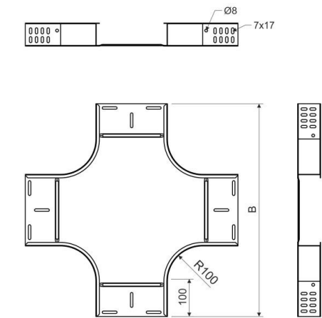
Maßzeichnung
