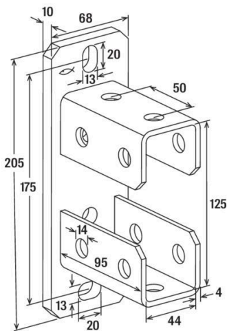
Maßzeichnung
