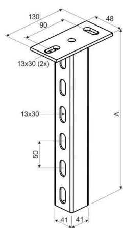
Maßzeichnung
