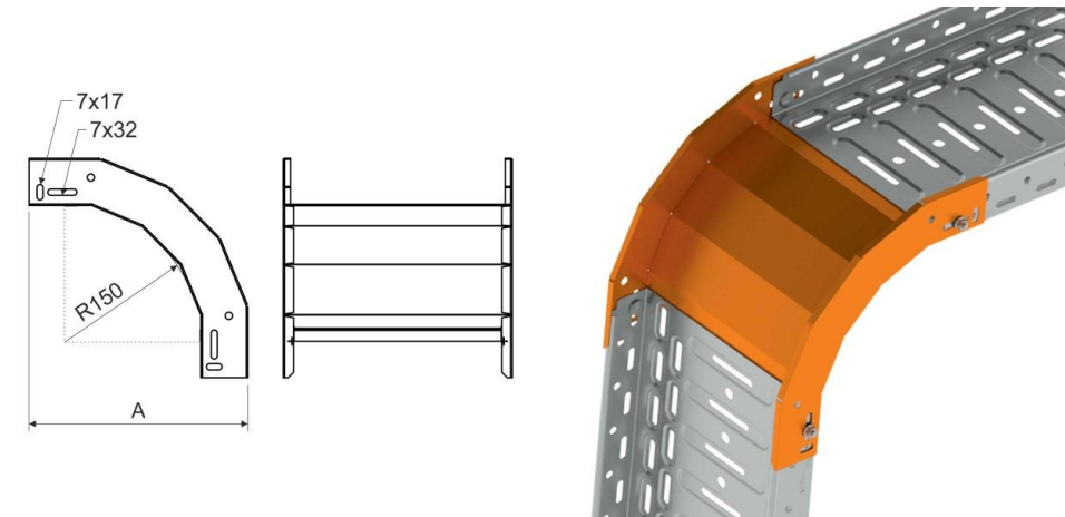
Maßzeichnung
